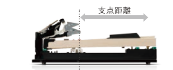
グランド・フィール・アクションⅢ
